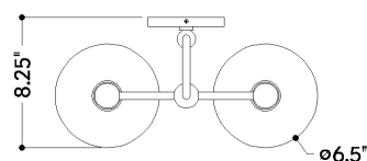
TOP
